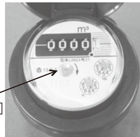
↑ 水道メータ（ふたを開けた状態）
